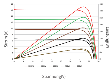
Strom-Spannungs- und Leistungs-Spannungs-Diagramme(445W)
